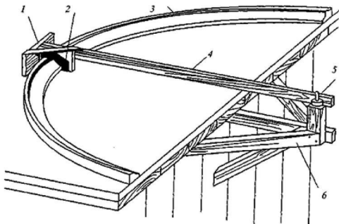
Рис. 7. Выполнение циркульной тяги: шаблон; 2 — углубление, препятствующее сдвигу слоев; 3 — салазки; 4 — направляющая; 5 — подкладка; 6 — выносная опора
