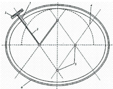
Рис. 8. Выполнение овальной тяги воробей-ножницами: 1 — полозок; 2 — радиусная рейка; 3 — упор; 4 — профильная доска; 5 — верстак; 6 — готовая тяга; 7 — линии разметки; 8 — центровой штифт
