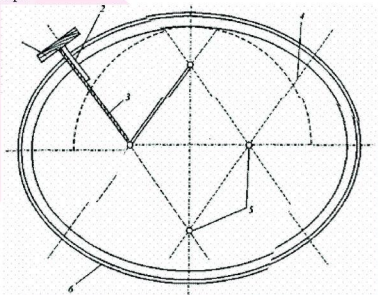
Рис. 9. Выполнение овальной тяги шаблоном на тесьме: 1 — полозок; 2 — профильная доска; 3 — тесьма; 4 — линии разметки; 5 — гвозди, забитые в центрах кривизны; 6 — готовая тяга
