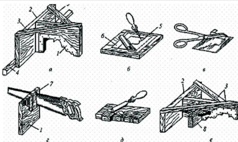
Рис. 3. Изготовления шаблона: а — готовый шаблон с одним полозком; б — перевод профиля на стальной лист; в — вырезание профиля; г — пропиливание профильной доски шаблона; д — выкалывание кусков между пропилами; е — готовый шаблон с двумя полозками; 1 — профильная доска с оковкой; 2 — доска-полозок; 3 — бруски-подкосы; 4 — направляющая рейка; 5 — чертеж профиля; 6 — лист металла; 7 — пропилены; 8 — второй брусок-полозок
