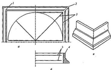
Рис. 5. Изготовление абакс дорической капители: а — план; б — разрез; в — склеенный угол; 1 — склеенный угол; 2 — приготовленный к склейке угол; 3 — арматура; 4 — профиль абакс.
