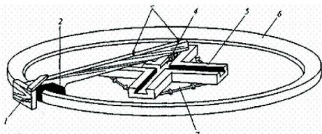
Рис. 10. Выполнение эллиптической тяги воробей и направляющим желобчатым патроном-крестом: 1 — полозок; 2 — шаблон-воробей; 3 — центровые штифты; 4 — челноки; 5 — патрон-крест; 6 — готовая тяга; 7 — листовая сталь
