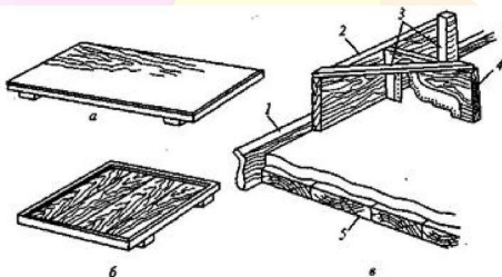
Рис. 2. Деревянные щиты для гипсового (а) и глиняного (б) грунта и шаблон для вытягивания прямолинейной гипсовой тяги карниза (в): 1 — направляющая рейка верстака; 2 — полозок; 3 — планки (расшивки); 4 — шаблон; 5 — верстак
