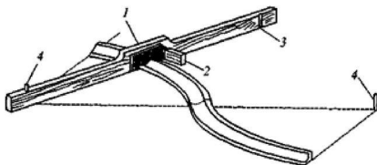
Рис. 11. Выполнение выпукло-вогнутой тяги: шаблон воробей; 2 — полозок; 3 — паз для центрового штифта; 4 — центральный штифт
